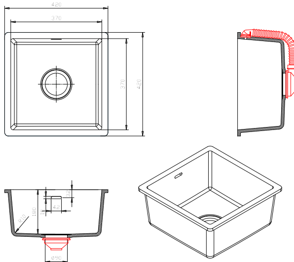
060 EMMA 370 mm / 370 mm / 180 mm / Ø 90 mm
