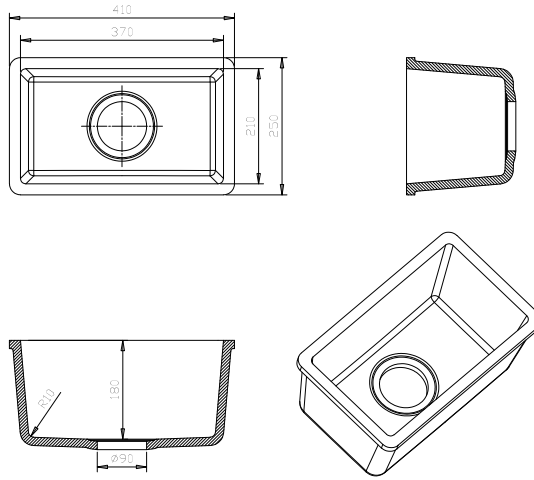
059 SONIA 370 mm / 210 mm / 180 mm / Ø 90 mm
