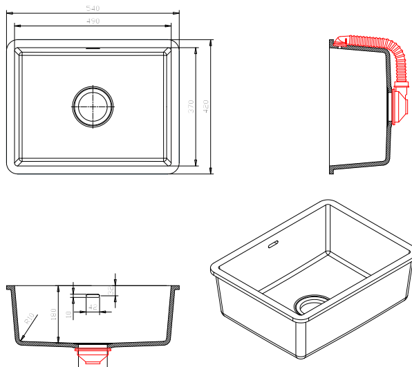
061 NADIA 490 mm / 370 mm / 180 mm / Ø 90 mm
