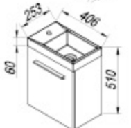
OUK 40 WH OUK 40 DO
